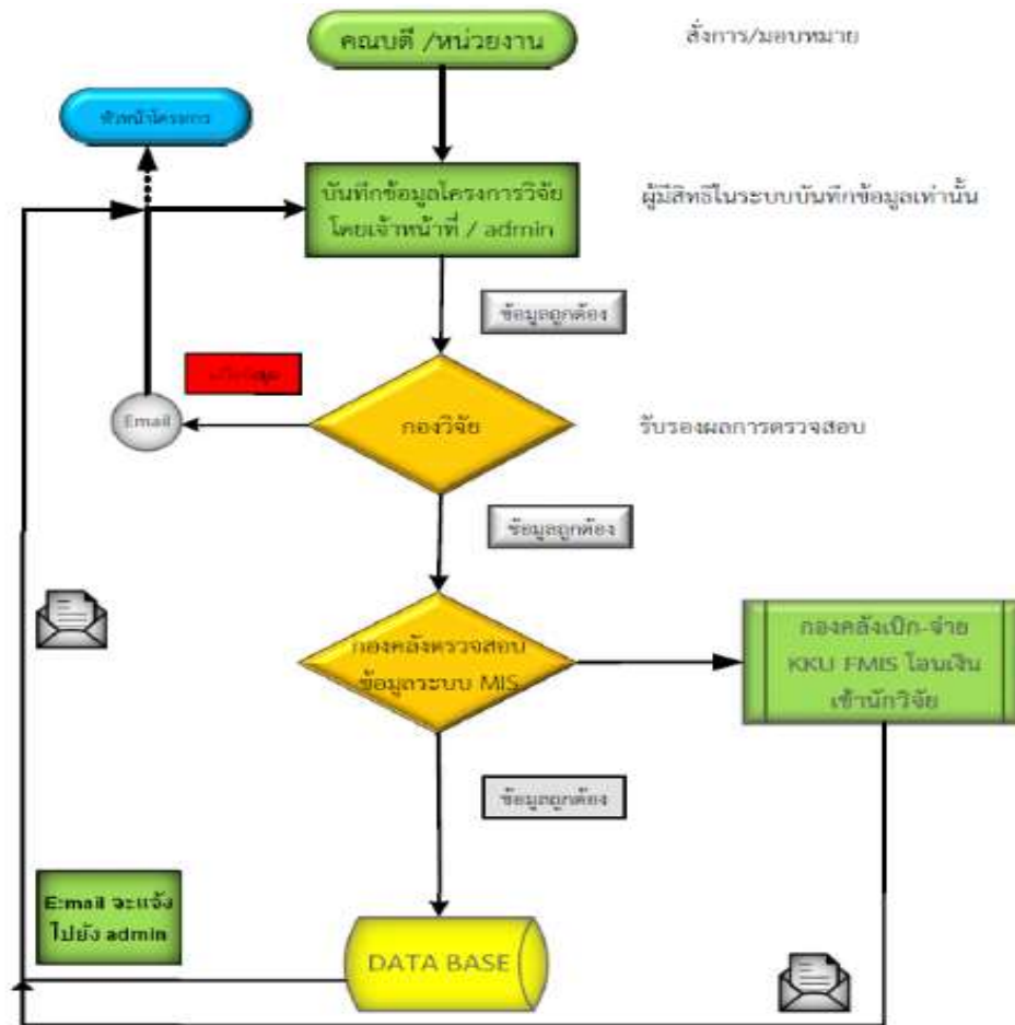
ภาพที่ 1.1 ขั้นตอนการดำเนินงานระบบ MIS KKU ( https://mis.kku.ac.th )
